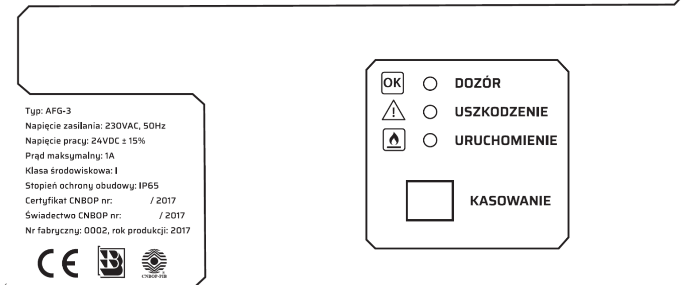
Rysunek 2. Panel sygnalizacyjno-kontrolny
