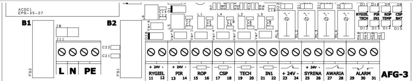
Rysunek 3. Pole przyłączeniowe
