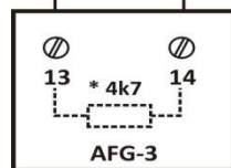
Rysunek 8. Podłączenie czujki dymu: MPD821 (CPD321), MMT860
