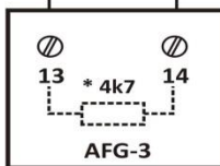
Rysunek 8. Podłączenie czujki dymu: MPD821 (CPD321), MMT860
