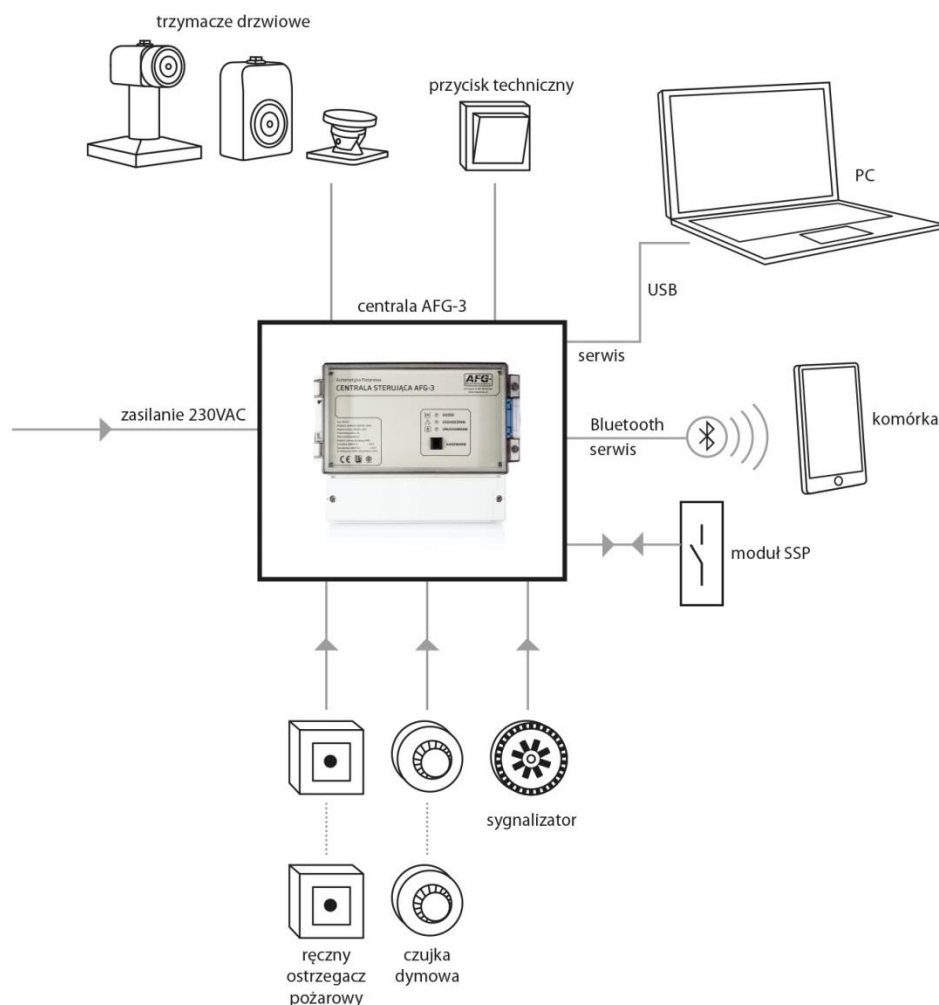
Rysunek 1. Schemat ogólny
