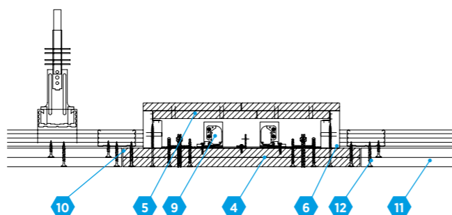
Detal A – Sposób montażu w suficie podwieszonym
