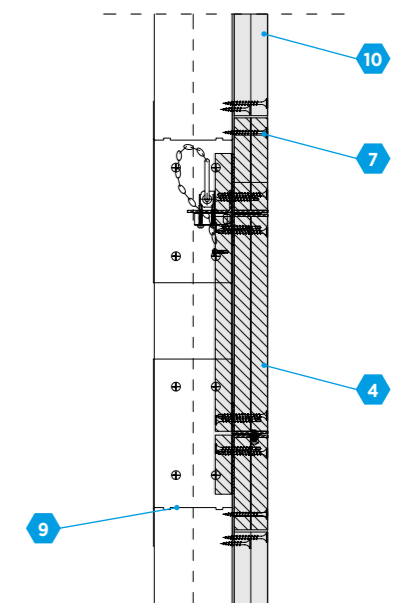
Detal A – Sposób montażu w ścianie g-k (przekrój)
