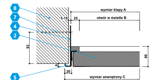
Detal C – Sposób montażu w ścianie masywnej
