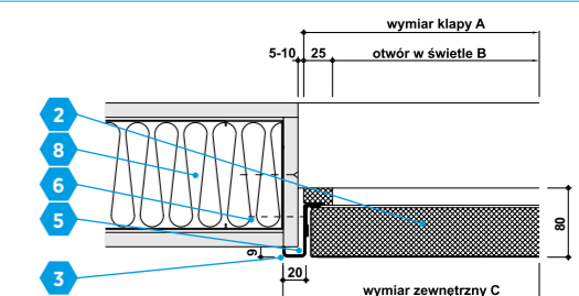
Detal B – Sposób montażu w ścianie lekkiej
