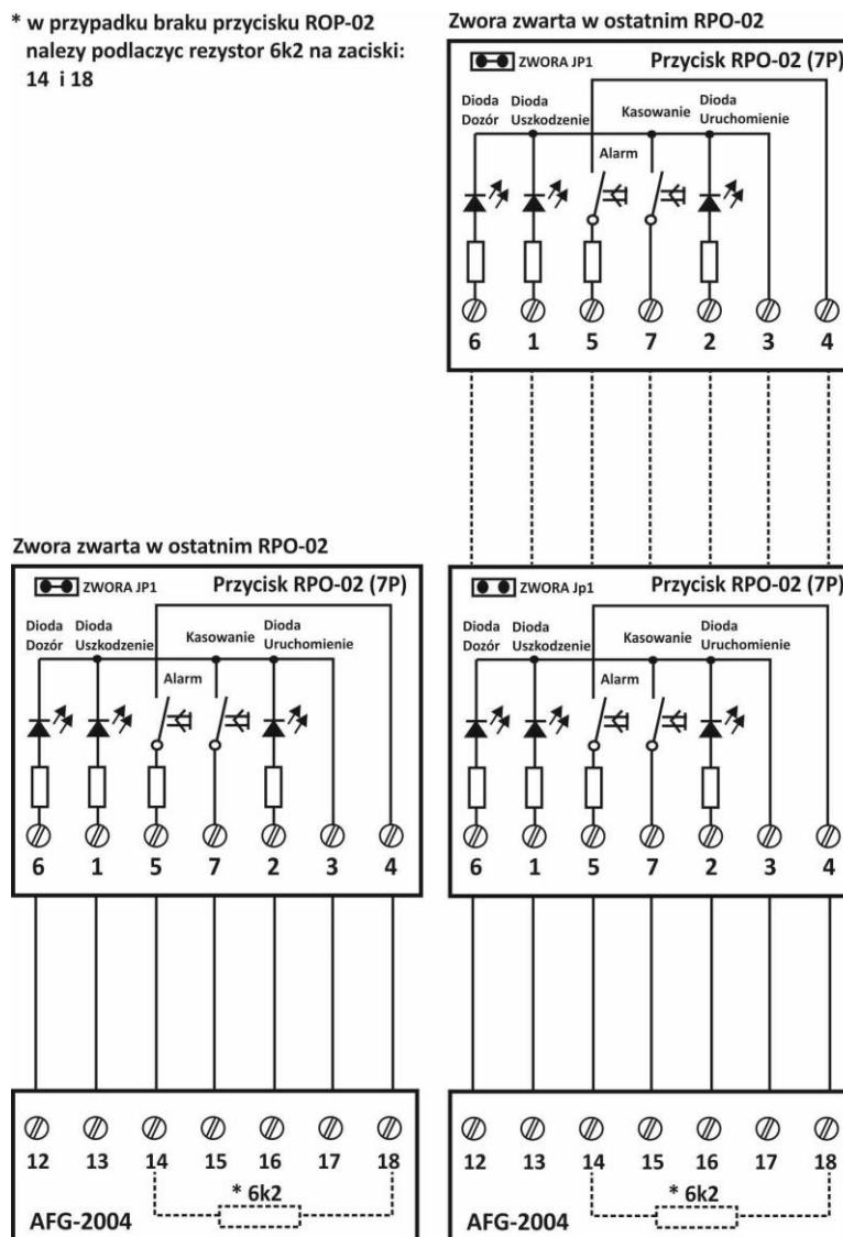
Rysunek 1. Schemat połączeń przycisku RPO-02/7P do centralki AFG-2004
