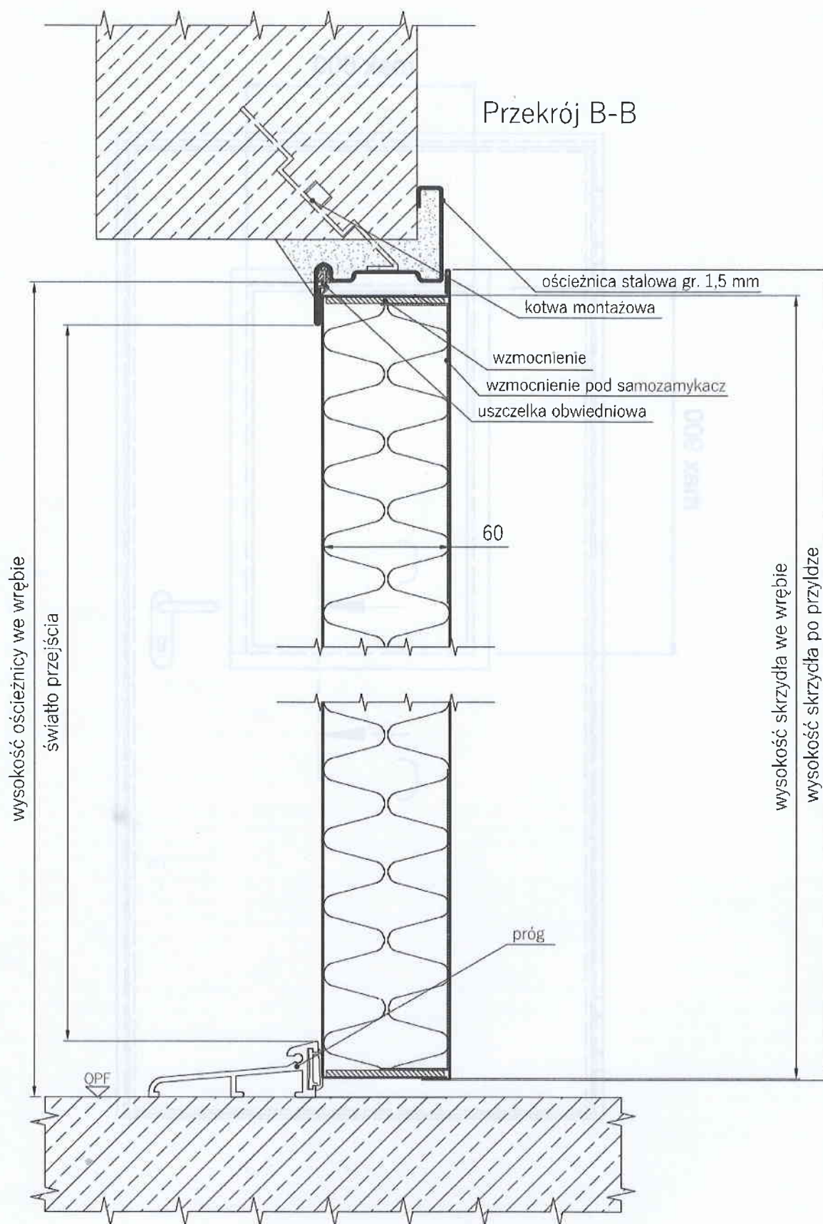
Rys. 31. Stalowe drzwi ENDOOR MULTI z przylgą wzdłuż krawędzi pionowych i górnej poziomej, z uszczelką przylgową oraz z progim z uszczelką – przekrój pionowy
