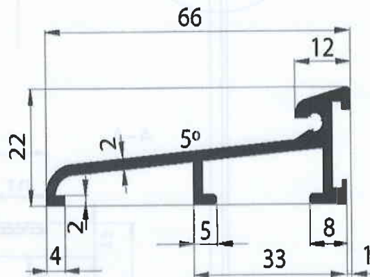
Rys. 37. Próg aluminiowy – przekrój
