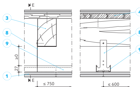
Przekrój B-B
