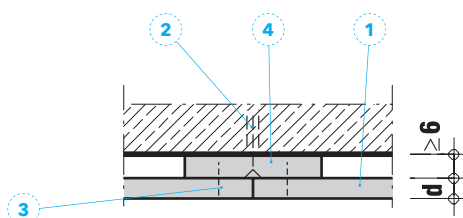
Detal B - Sposób montażu
