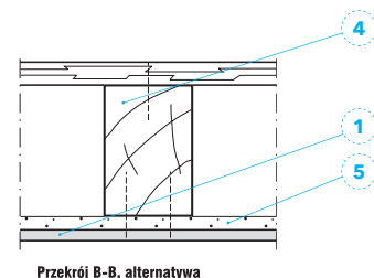
Przekrój B-B, alternatywa
