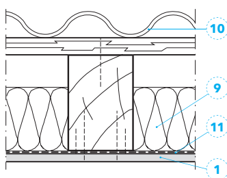
Przekrój B-B
