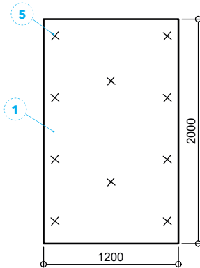
Detal B - Rozkład placków kleju
