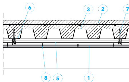
Detal B - Przekrój podłużny
