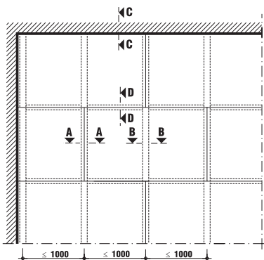
Detal A - Widok stropu
