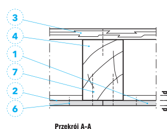
Przekrój A-A
