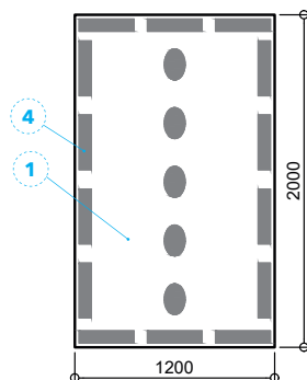
Detal B - Rozkład placków kleju
